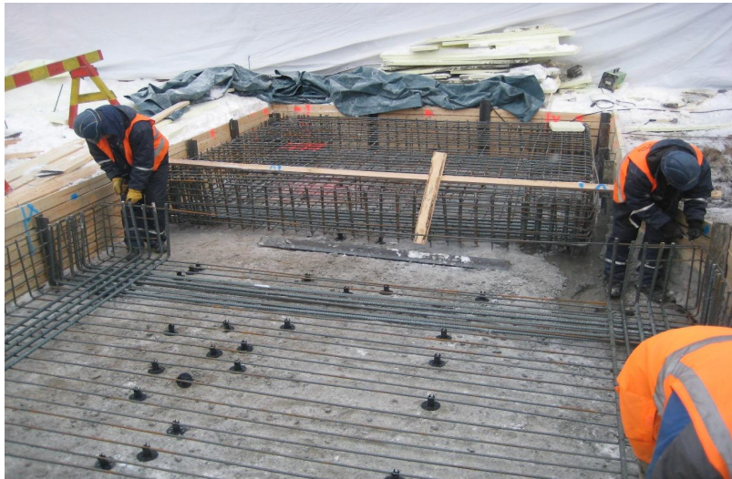
Hissin pohjalaatan raudoitustyö käynnissä.
